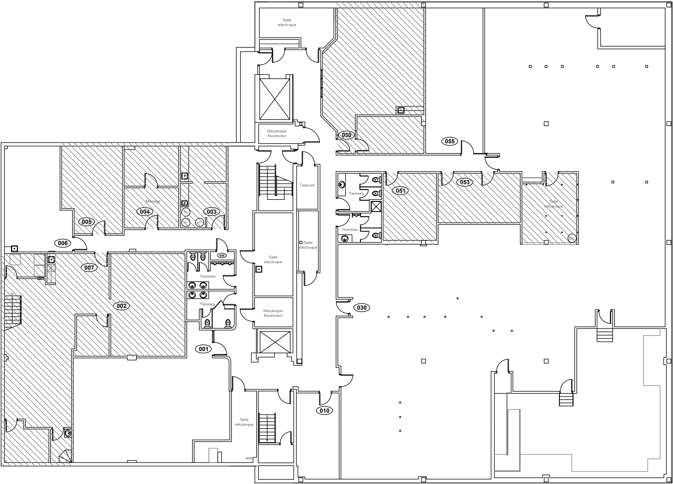
Sous-sol
